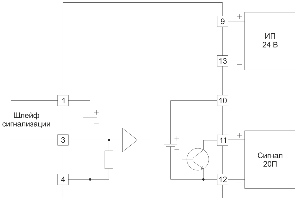
Схема использования в шлейфе сигнализации (ШС) на примере ШС «Сигнал 20П»
