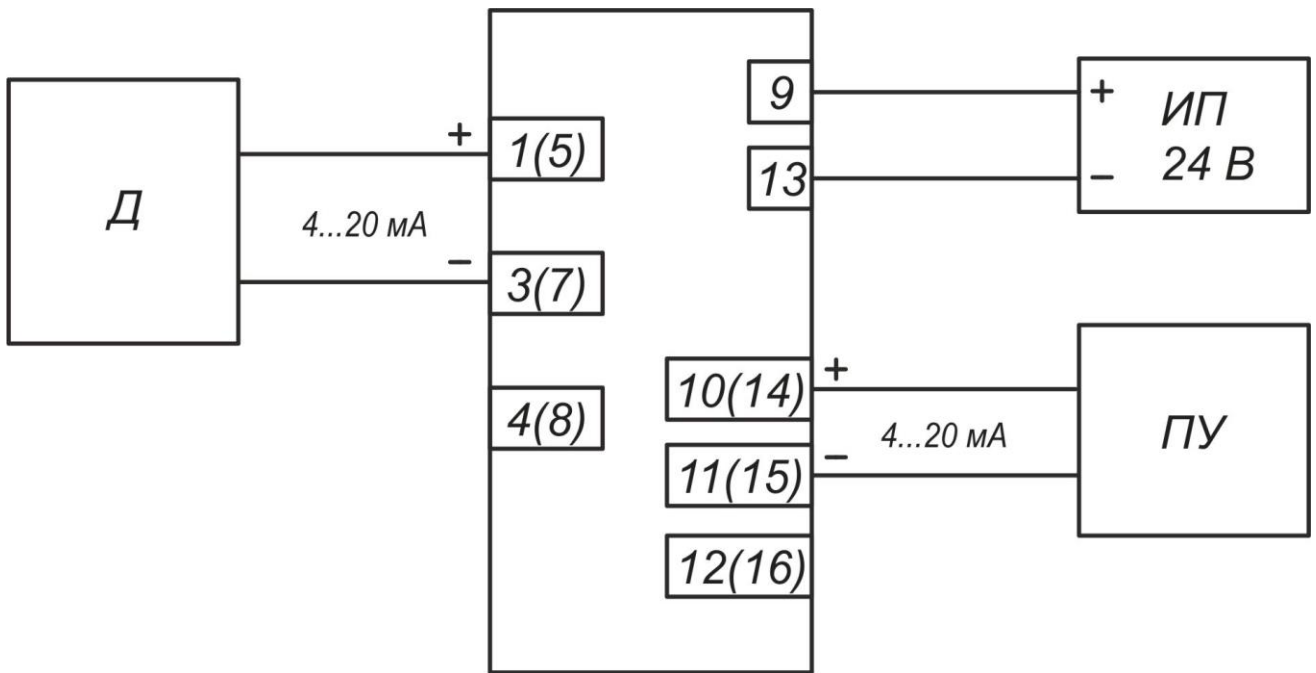
Схема подключения барьеров НБИ-ХОП
