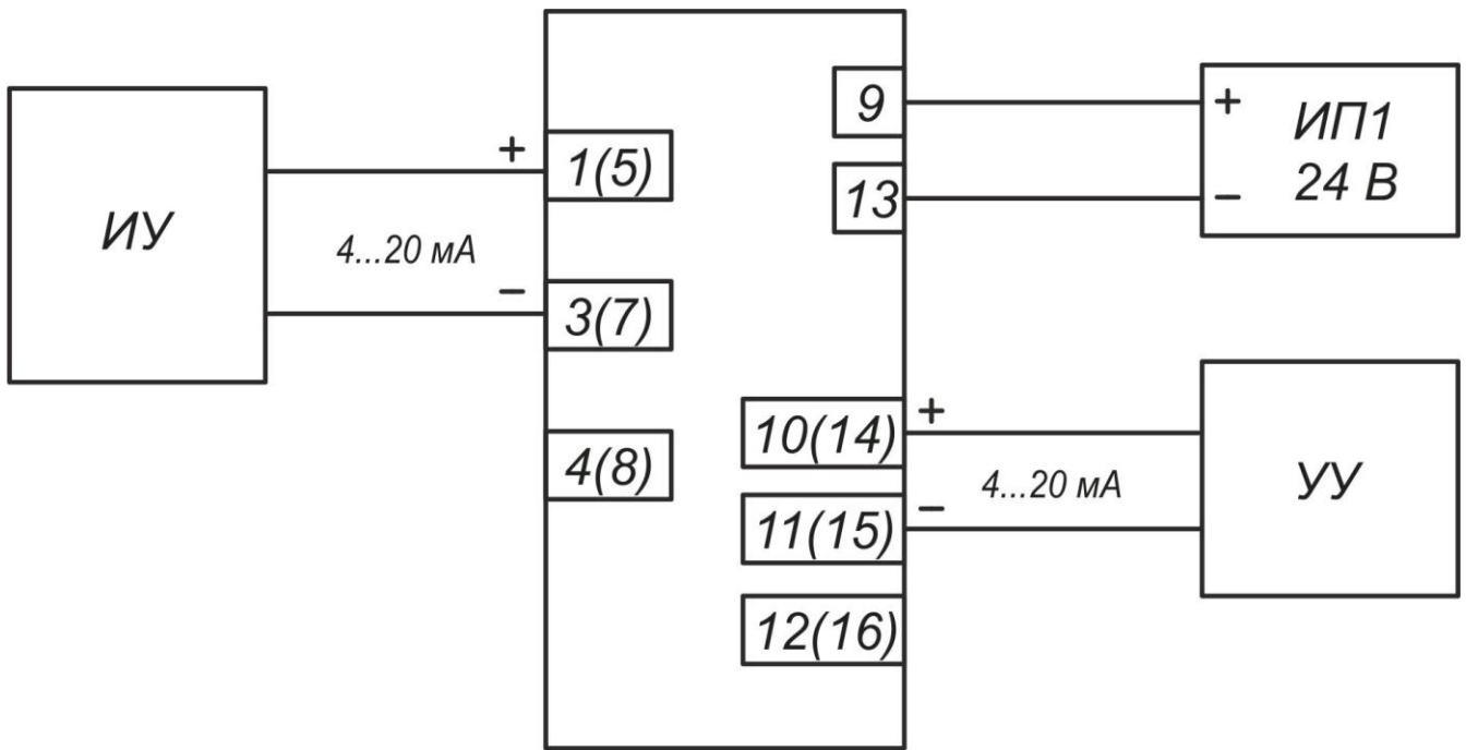
Схема подключения барьеров НБИ-Х0У
