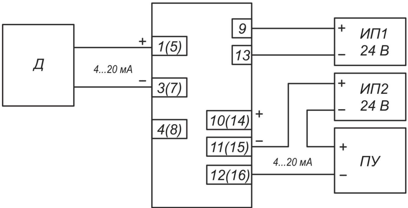
Схема подключения барьеров НБИ-Х1П
