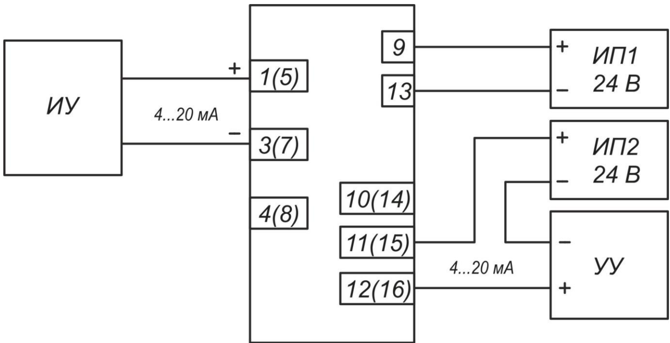
Схема подключения барьеров НБИ-Х1У
