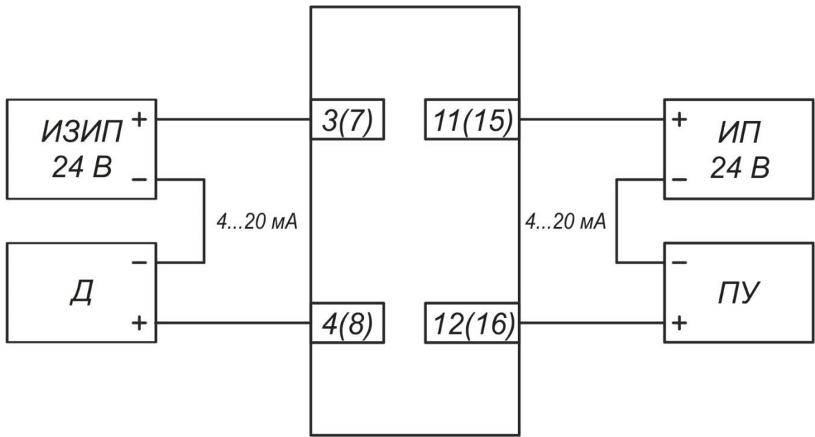
Схема подключения барьеров НБИ-Х2П
