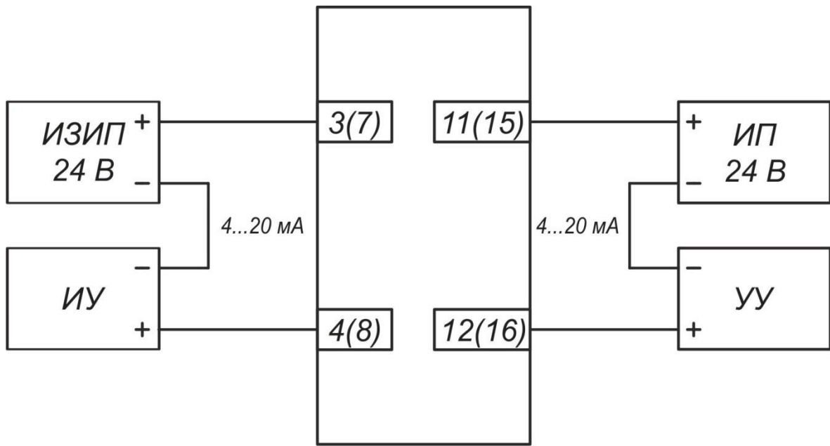
Схема подключения барьеров НБИ-Х2У
