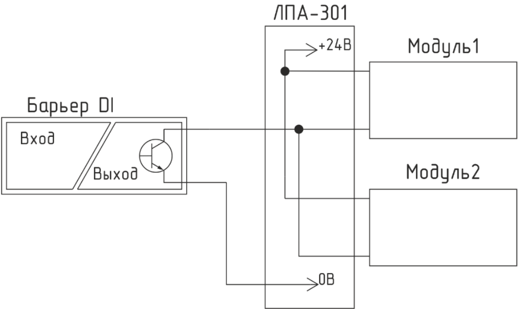
Рисунок 1 – Схема резервирования входного дискретного сигнала типа «открытый коллектор» с общим плюсом
