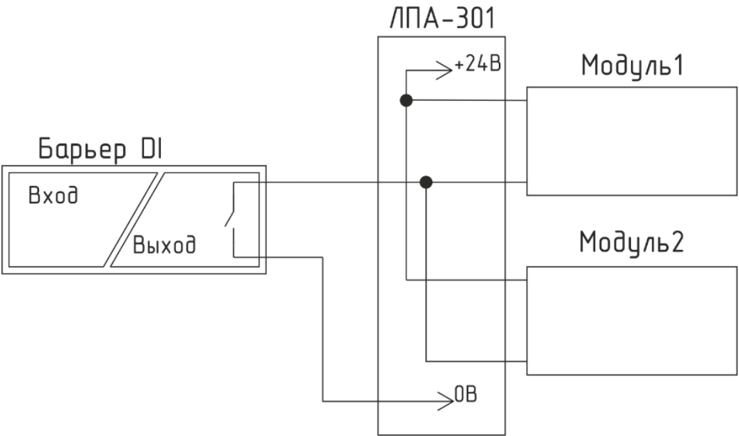
Рисунок 1 – Схема резервирования входного дискретного сигнала типа «открытый коллектор» с общим плюсом
