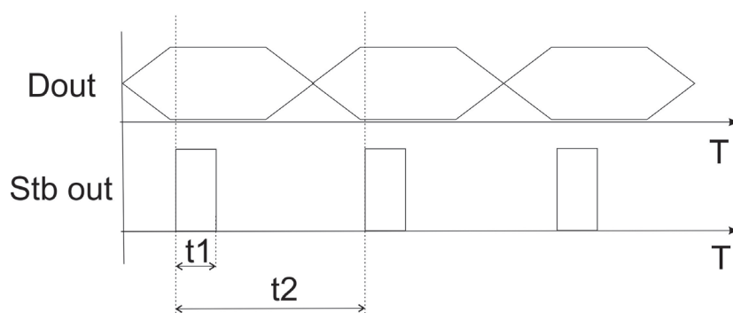
Рис. 8. Временная диаграмма синхроимпульсов для исходящих сигналов
