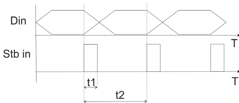
Рис. 7. Временная диаграмма синхроимпульсов для входящих сигналов
